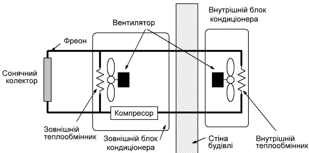
Рис. 3. Підключення сонячного колектора до кондиціонера
