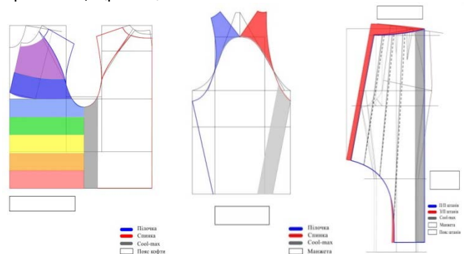
Рис. 4. Кресленник МК основи кофти, рукава реглан та штанів-афгані
