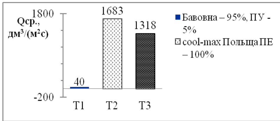
Рис. 1. Гістограми значень повітропроникності трикотажних полотен
