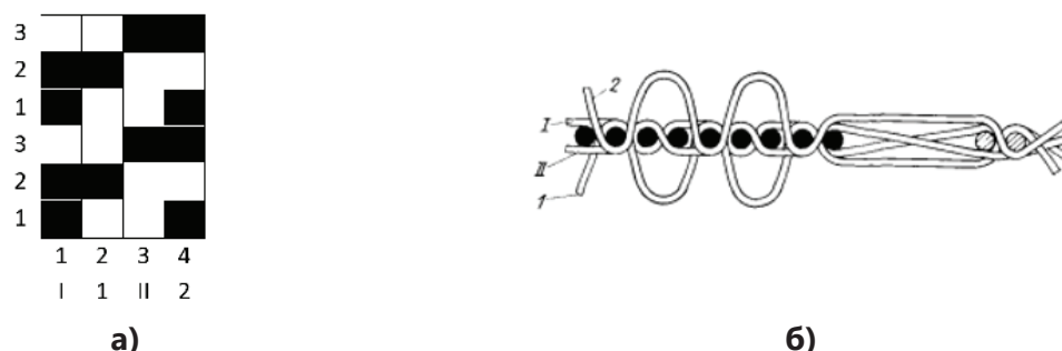
Рис.2. Махрова тканина: а – рисунок переплетення; б – переріз тканини
