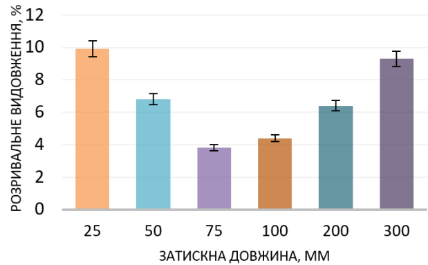
Рис. 2. Діаграми розривального зусилля (а) та видовження (б) при заправці у затискачі 6 pA ниток лінійної густини 44 текс
